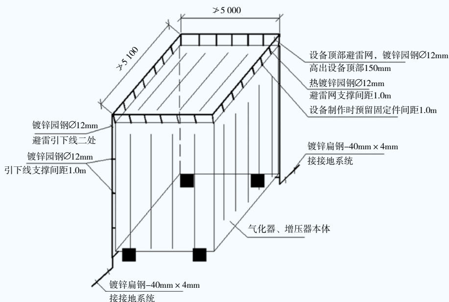
图1 气化器、增压器顶部安装避雷网示意图
