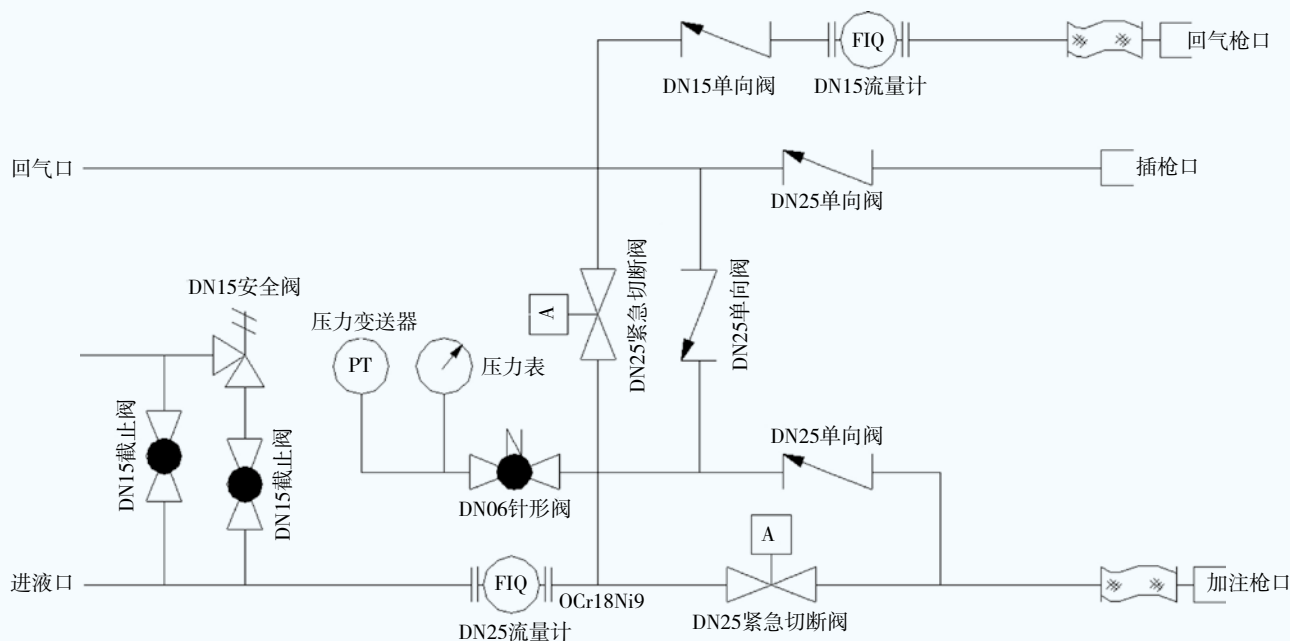
图1 LNG加注机工艺流程图
